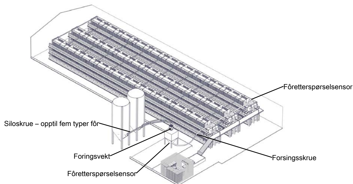
6: Skjematisk tegning av egglegger-fôringssystem for et bursystem.
