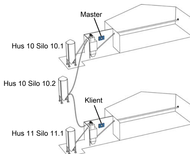
15: Eksempel på silo delt mellom to hus med kontrollere på LAN.
