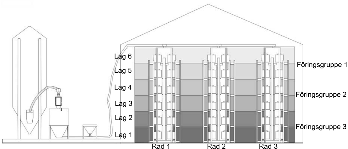
7: Betegnelser som gjelder foring for eggleggende i et bursystem.
